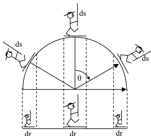
Fig. 2. Gekrümmte Raumzeit im Gegensatz zu Maßstabsveränderungen im Gravitationsfeld.
