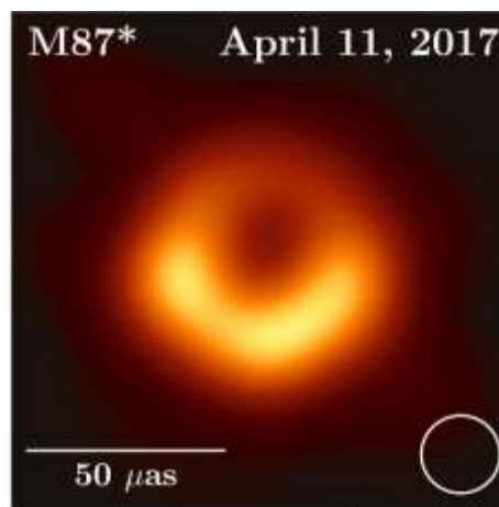
Fig. 1. Das erste Foto eines schwarzen Lochs.
